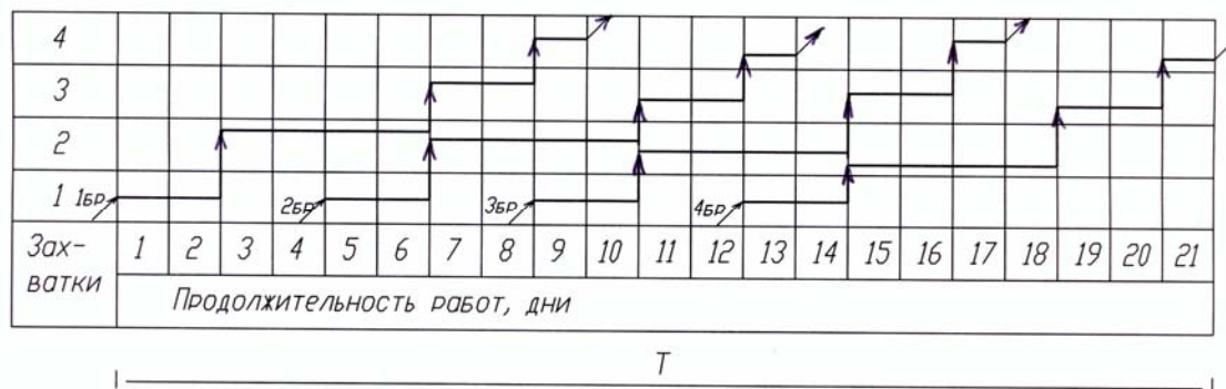
Рисунок 9 – Линейный график (а) и циклограмма (б) специализированного неритмичного потока с однородным изменением ритма
