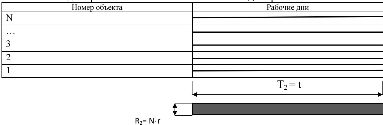
Рисунок 2 - Линейный график строительства N одинаковых объектов параллельным методом
