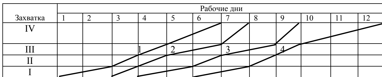
Рисунок 13 – Циклограмма неритмичного потока с неоднородным изменением ритма
