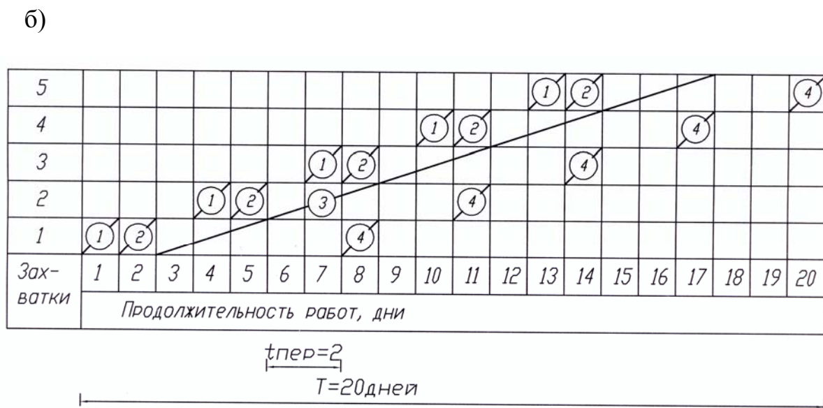
Рисунок 8 – Линейный график (а) и циклограмма (б) специализированного кратноритмичного потока при уравнивании его по замедленному ритму
