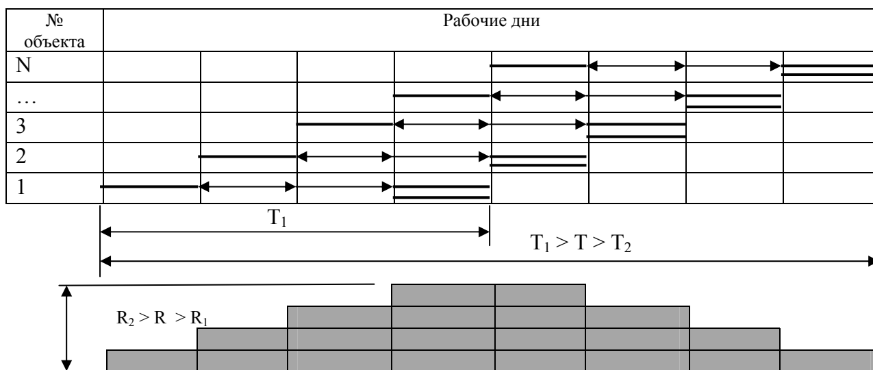
Рисунок 3 – Линейный график строительства N одинаковых объектов поточно-расчлененным методом
