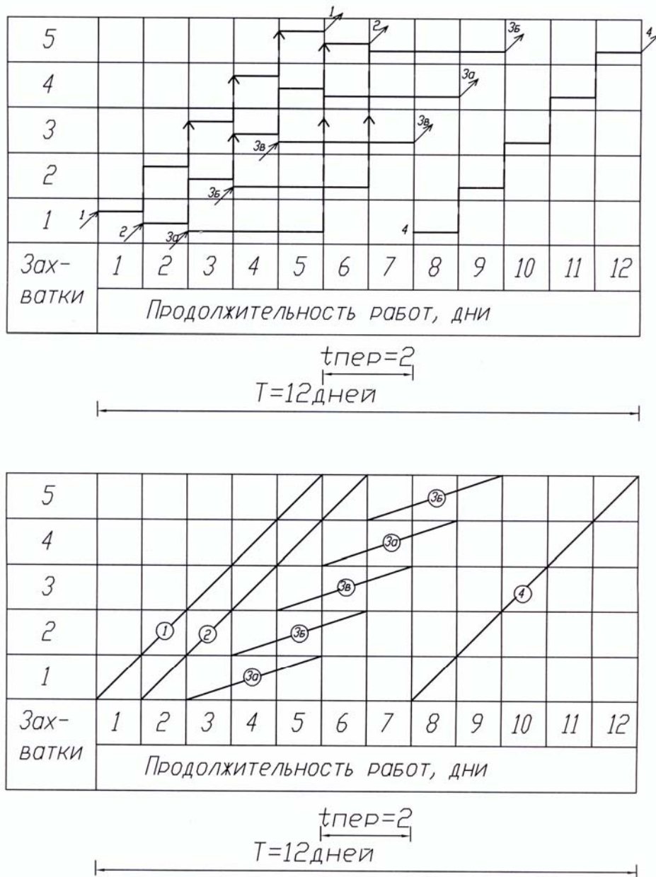
Рисунок 7 – Линейный график (а) и циклограмма (б) специализированного потока при уравнивании его по ускоренному ритму
