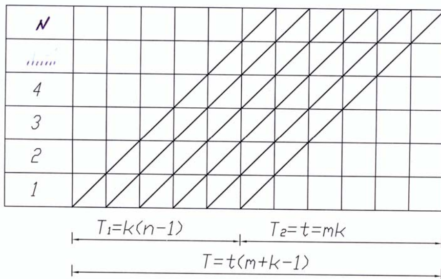
Рисунок 4 – Циклограмма строительного потока
